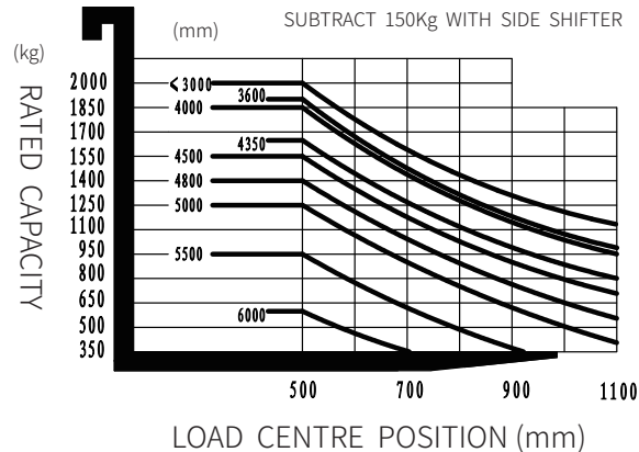
ГРАФИК НОМИНАЛЬНОЙ ГРАЗПОДЪЕМНОСТИ
