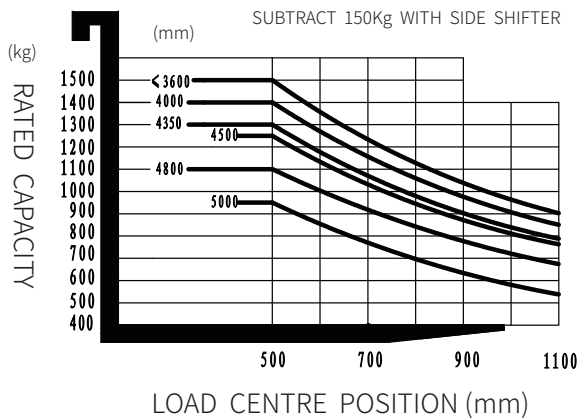
ГРАФИК НОМИНАЛЬНОЙ ГРАЗПОДЪЕМНОСТИ
