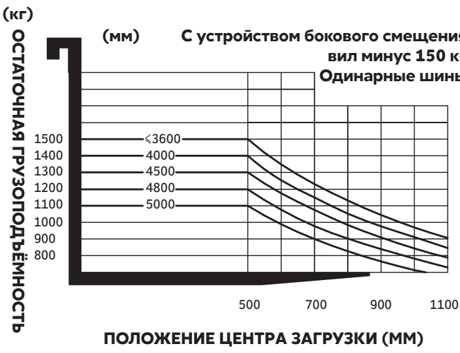
График падения грузоподъёмности CPD15TVL
