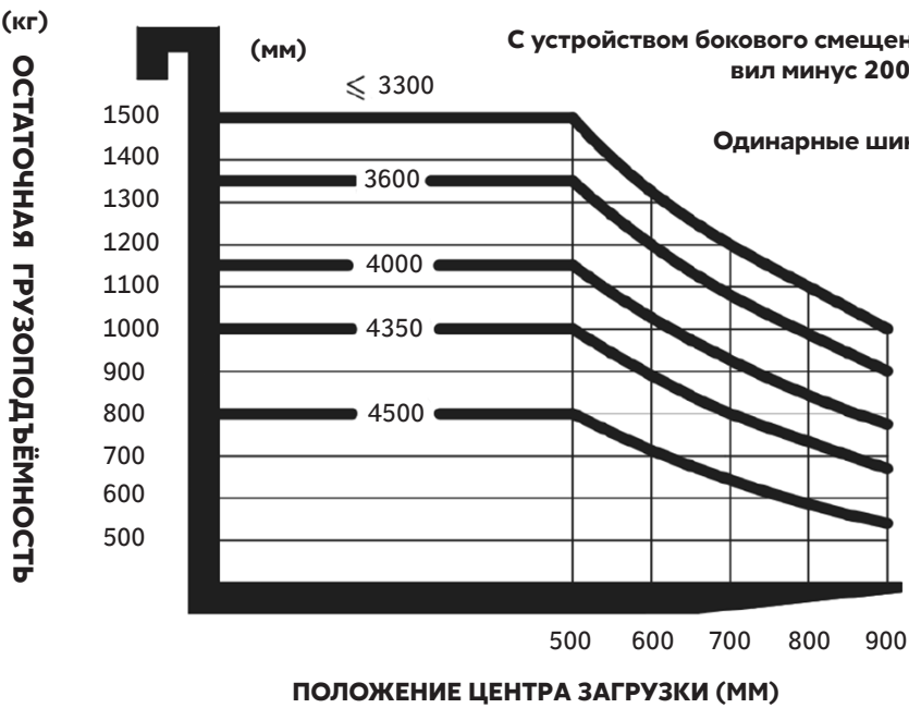
График остаточной грузоподъёмности EFS151
