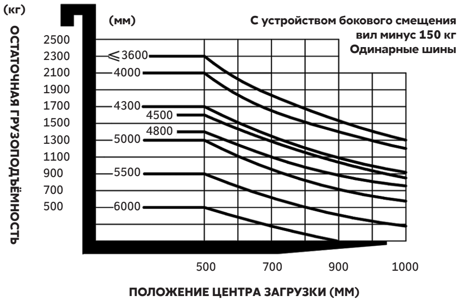
График падения остаточной грузоподъёмности EFL252
