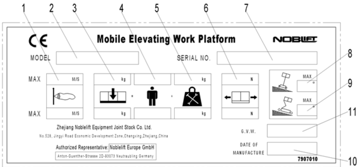
Рис. 3-4. Идентификационная табличка.
